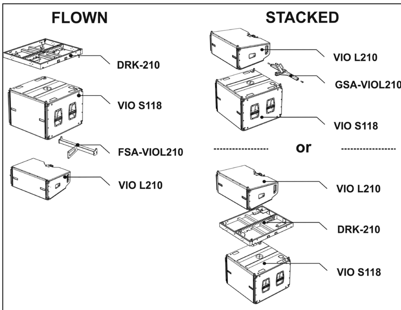
Verwendungsschema des Montagezubehörs
