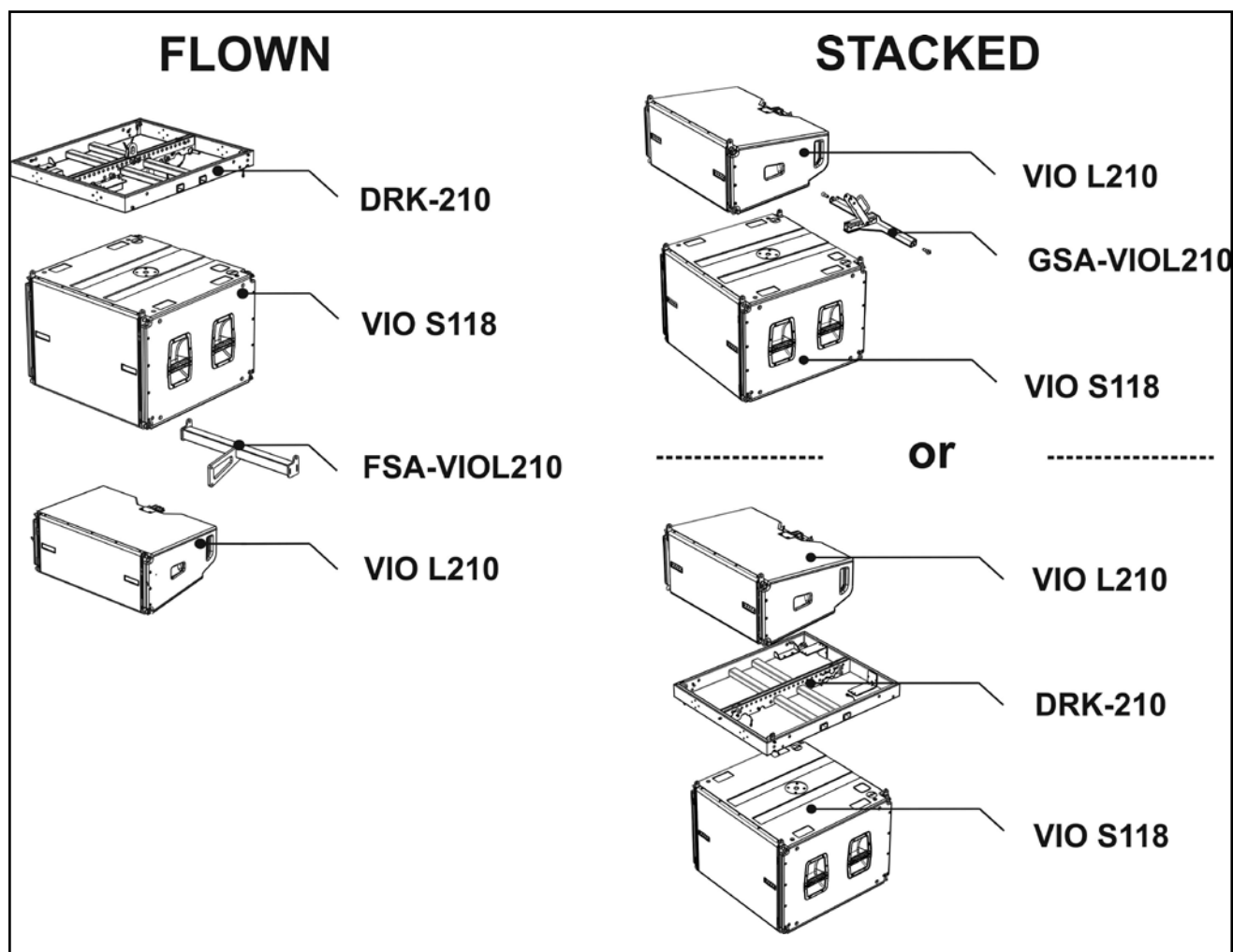
Schema di utilizzo degli accessori di montaggio
